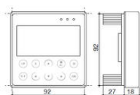
DIRIS Digiware D-40/D-50/D-70
