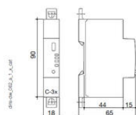
DIRIS Digiware C-31
